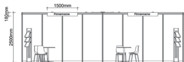
Vorderansicht
