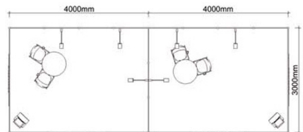
Grundriss
